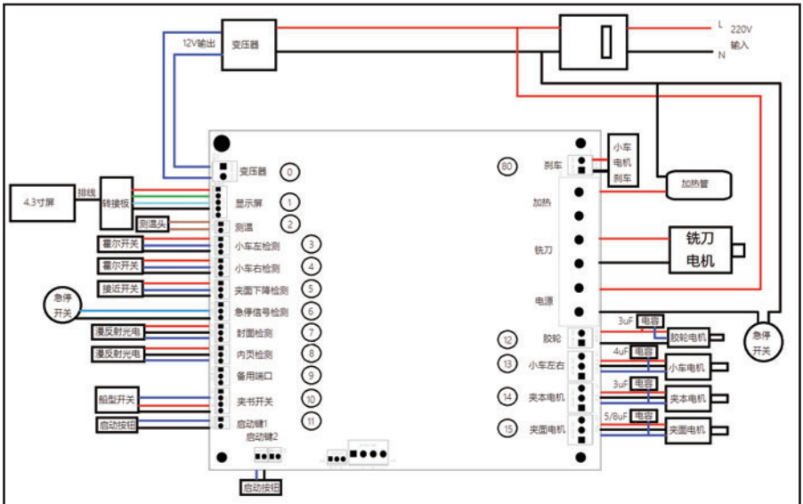
336C线路图
